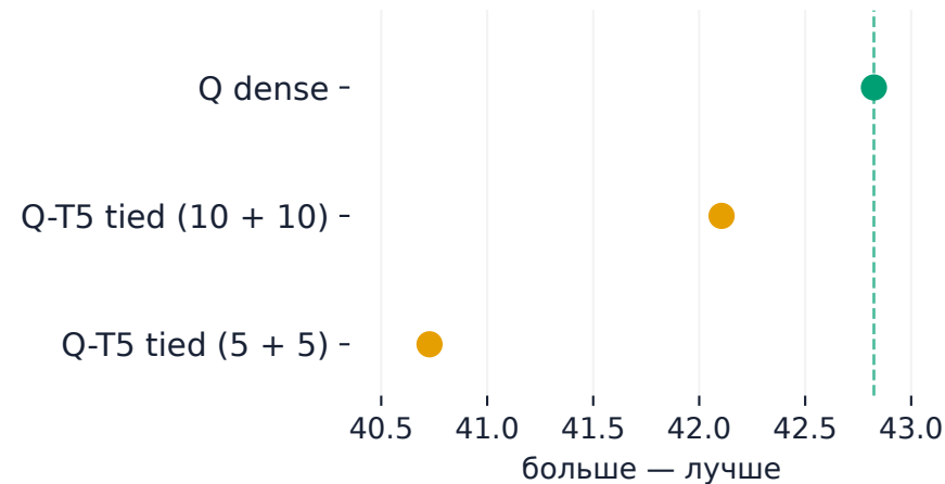
Среднее задач, %
