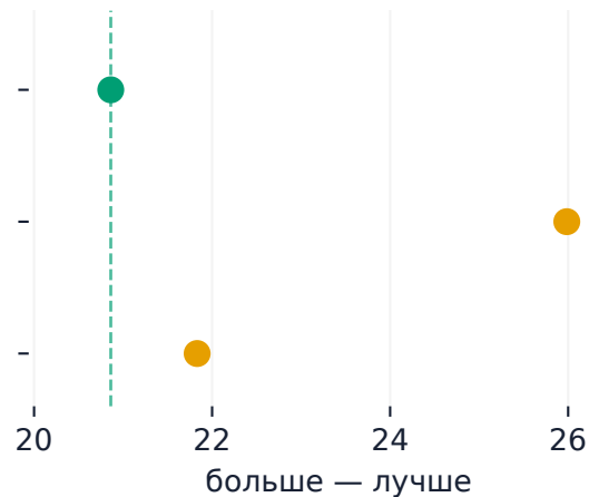
LAMBADA, %
